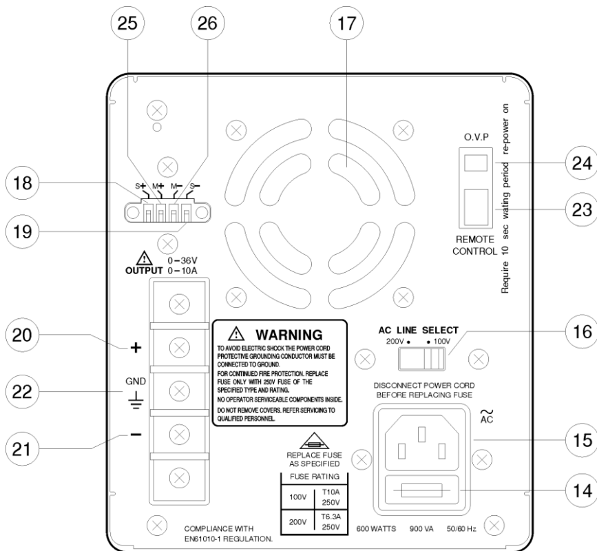
図 4-2 リアパネル
