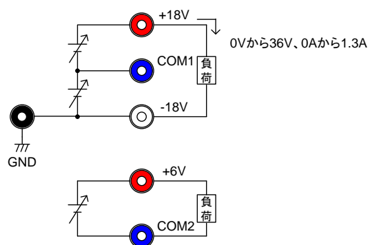
図 7-4. 直列接続
