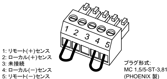
図 2-7 センシング接続の初期設定
