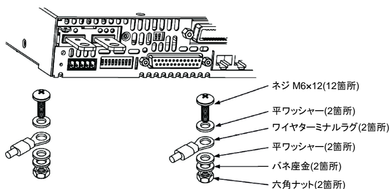
図 2-8 負荷線の接続方法(6V~60V 出力電圧モデル)
