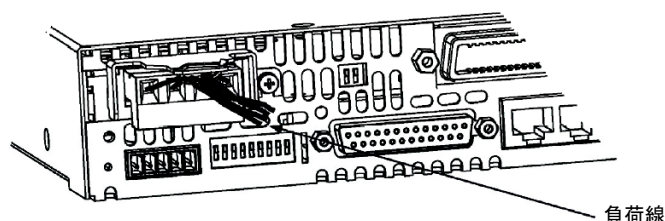
図 2-12 保護カバーと負荷線の取付け
