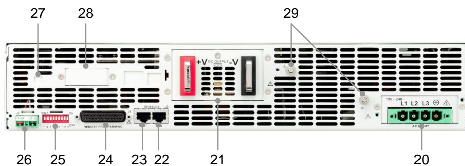
図 3-7 3300W / 5000W リアパネルコネクタ
