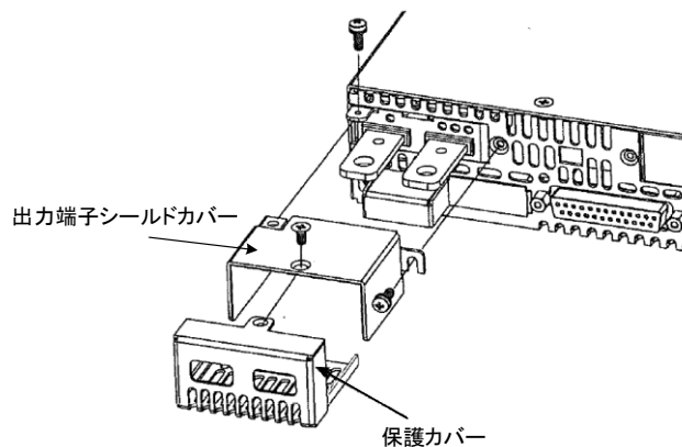
図 2-9 出力端子用シールドカバーの取付け
