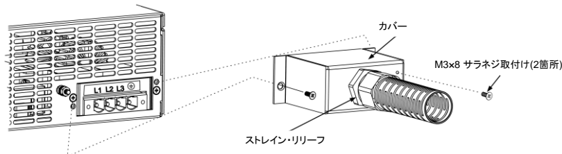
図 2-6 AC 入力カバーの取付け
