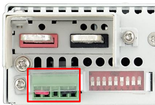
図 2-27 750W センシング端子図
