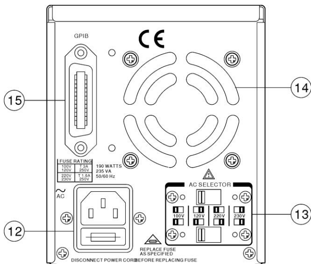
図 4-2 リアパネル
