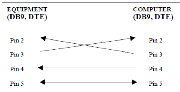
図 2 DB9 から DB9 への配線接続(GTL-232A)
