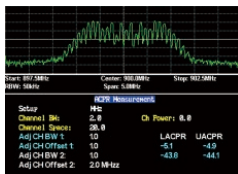
ACPR測定
