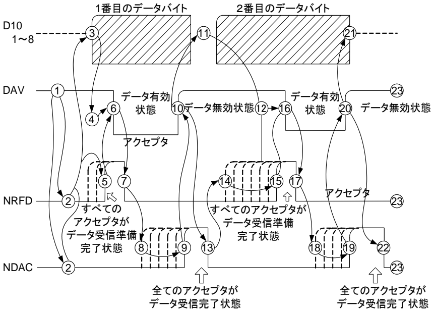
ハンドシェイクシーケンスのタイミングチャート
