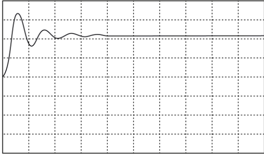
ARB11 2次ステップ応答(減衰係数 0.7)
